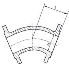
Łuki dwukołnierzowe FFK 11/22/30/45 stopni nr 9209 żeliwo sferoidalne GGG40
