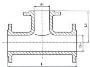
Trójnik kołnierzowy T nr 9203 żeliwo sferoidalne GGG40
