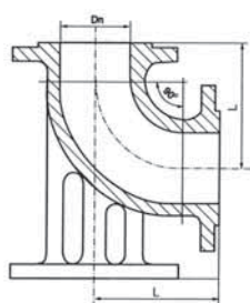
Kolano kołnierzowe ze stopką N nr 9202 żeliwo sferoidalne GGG40
