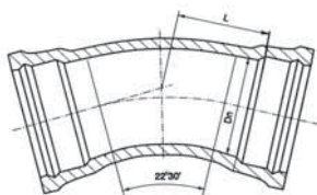
Łuki dwukielichowe MMK 11/22/30/45 st. nr 9210 żeliwo sferoidalne GGG40
