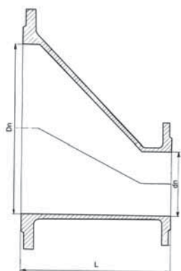
Zwężka dwukołnierzowa asymetryczna FFRE nr 9213 żeliwo sferoidalne GGG40
