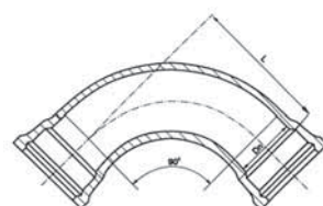
Kolano dwukielichowe MMQ 90 nr 9208 żeliwo sferoidalne GGG40
