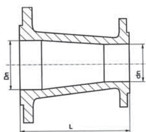
Zwężka dwukołnierzowa FFR nr 9212 żeliwo sferoidalne GGG40
