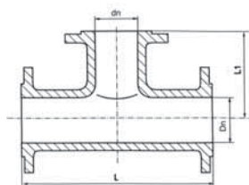
Trójnik kołnierzowy T nr 9203 żeliwo sferoidalne GGG40
