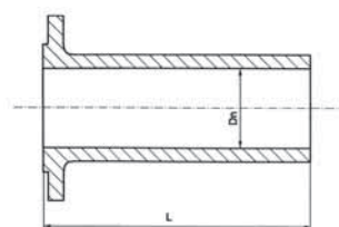
Króciec jednokołnierzowy F nr 9201 żeliwo sferoidalne GGG40
