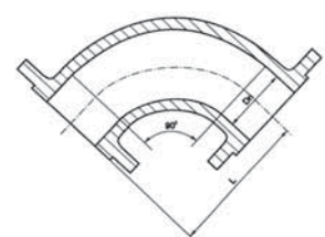
Kolano dwukołnierzowe Q 90 nr 9207 żeliwo sferoidalne GGG40
