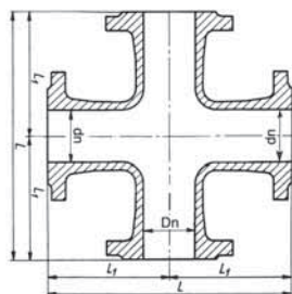
Czwórnik kołnierzowy TT nr 9218 żeliwo sferoidalne GGG40
