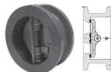
Zawór zwrotny motylkowy nr 6535, dysk AISI 316
