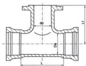
Trójnik kielichowo-kołnierzowy MMA nr 9205 żeliwo sferoidalne GGG40
