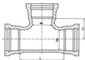
Trójnik trzykielichowy MMB nr 9206 żeliwo sferoidalne GGG40
