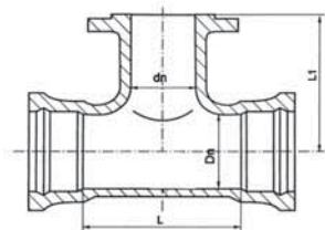
Trójnik kielichowo-kołnierkowy MMA nr 9205 żeliwo sferoidalne GGG40
